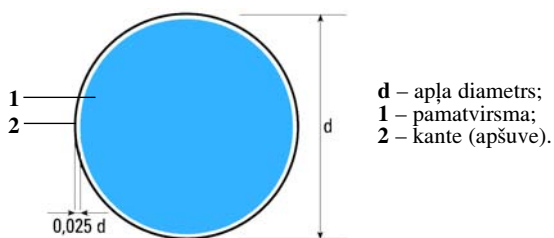
3. attēls. Rikojuma zīmju krāsu grafiskais attēlojums un izmēru attiecība
