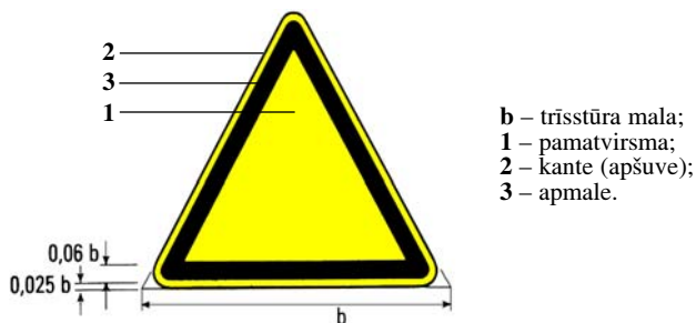
2. attēls. Bīdinājuma zīmju krāsu grafiskais attēlojums un izmēru attiecība
