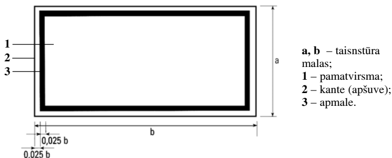
6. attēls. Informācijas zīmju krāsu grafiskais attēlojums un izmēru attiecība
