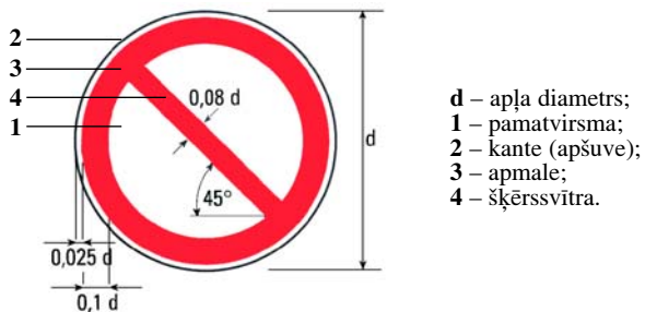
1. attēls. Aizlieguma zīmju krāsu grafiskais attēlojums un izmēru attiecība
